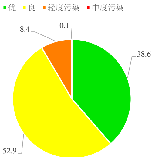
图1 2023年5月浙江省县级及以上城市日空气质量统计
