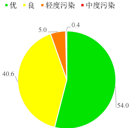
图1 2023年8月浙江省县级及以上城市日空气质量统计
